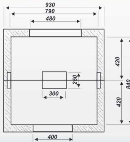
Przekrój poprzeczny
